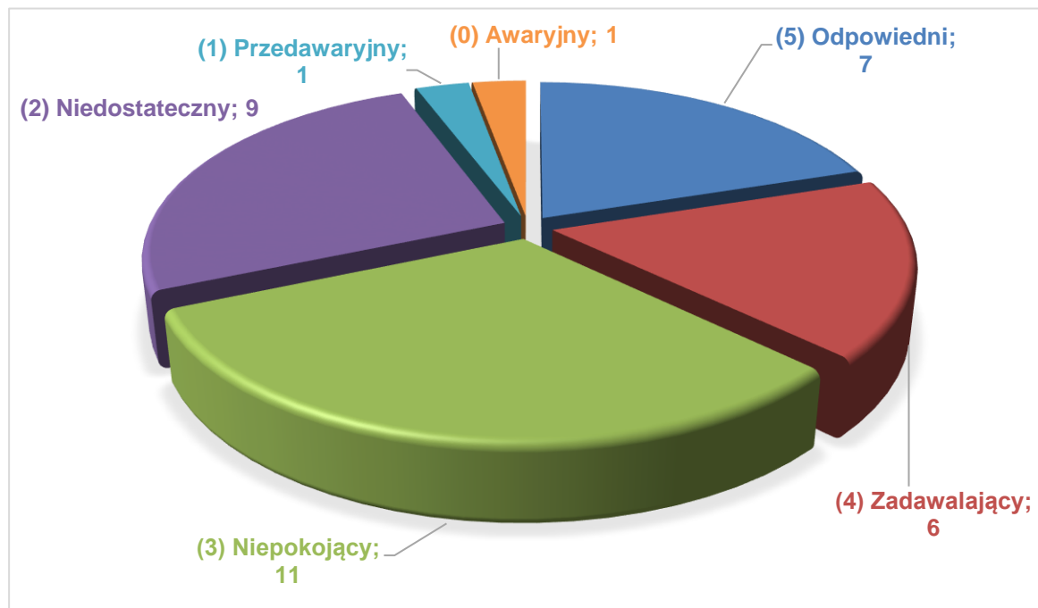
Wykres 7: Stan techniczny obiektów mostowych
